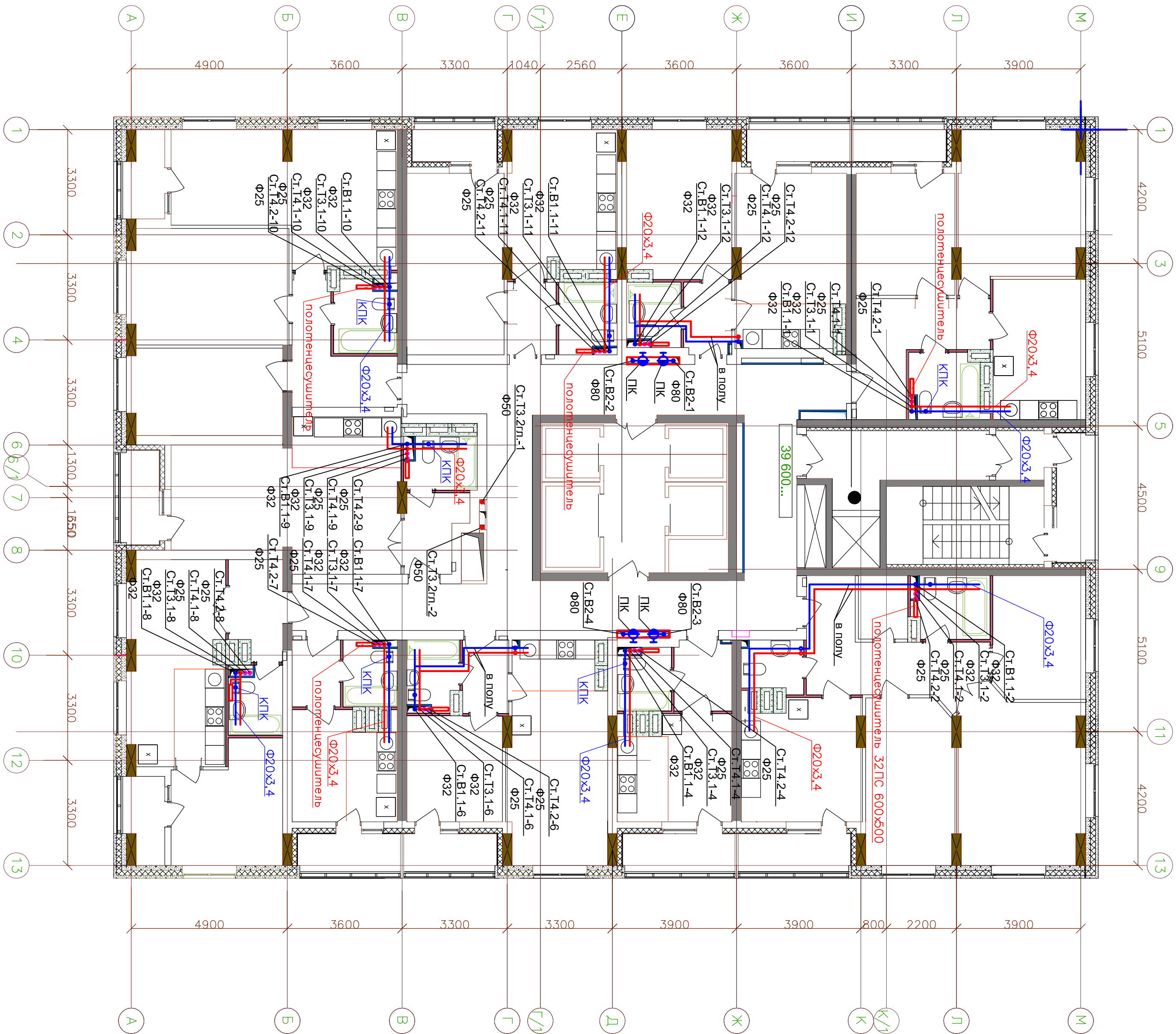
План 14 этажа с сетями В1.1, В2, Т3.1, Т3.2, Т4.1, Т4.2
